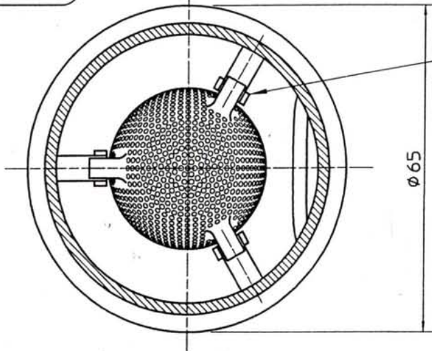
Schnitt A-A
